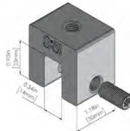
S-5!® S-Mini
