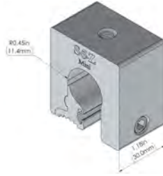
S-5!® Z-Mini
